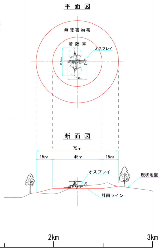
ヘリコプター着陸帯平面及び断面形状
